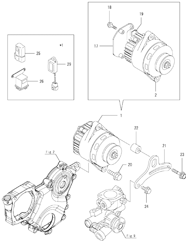
Fig.15. GENERATOR
