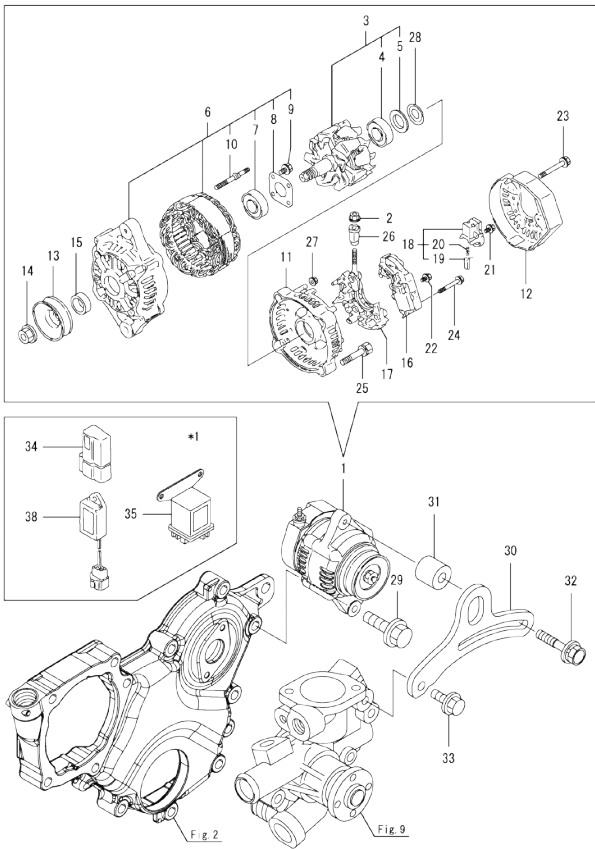
Fig.17. (15A)GENERATOR
